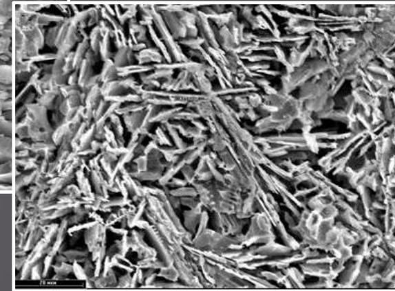
Форма первинних кристалів і морфологія евтектики сплаву Al-18%Si
