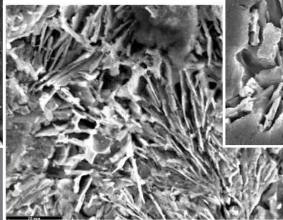
Форма первинних кристалів і морфологія евтектики сплаву Al-18%Si
