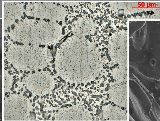
Структура сплаву Al-7%Si
