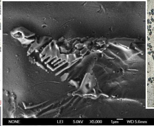
Структура сплаву Al-7%Si
